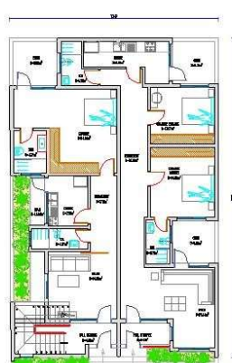
01_VUE EN PLAN REZ DE CHAUSSEE
